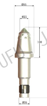
FZ-U170-25
