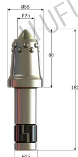
FZ-U95-25
