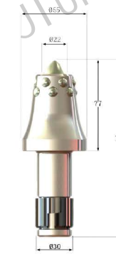
FZ-U84-22
